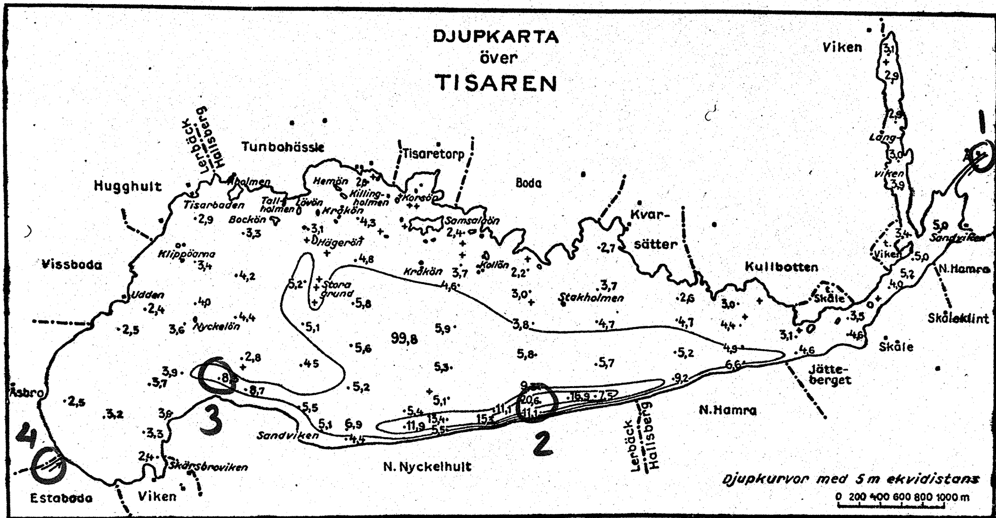
Fig. 2. Djupkarta över Tisaren, lodad från isen vårvintern 1926. Tisarens raka södra strand bestämmes av en brottlinje från Viken i väster till Skåle i öster. Brottzonen är av isen nederoderad till en ränna, som i sjön är upp till 21 meter djup men i väster, vid Sandviken, går upp på land och där avskär det i sjön utskjutande Fyrnäsberget. 160 lodskott från isen, av vilka endast ett urval är medtaget.
